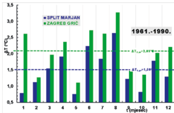
Slika 6: Histogrami mjesečnih razlika, \Delta T = T - T_{pr} , Split Marjana (modra boja) i Zagreb Griča (zeleno) u posljednjih deset godina (2011. - 2020.) u odnosu na prvo 30-godišnje razdoblje (1961. - 1990.)
