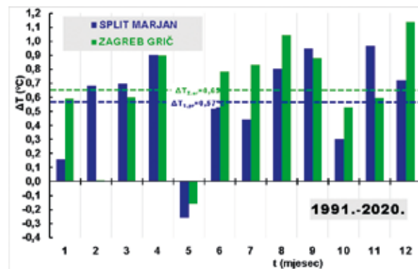
Slika 9: Histogrami mjesečnih razlika, \Delta T = T - T_{pr} , Split Marjana (modra boja) i Zagreb Griča (zeleno) u posljednjih deset godina (2011. - 2020.) u odnosu na četvrto 30-godišnje razdoblje (1991. - 2020.)
