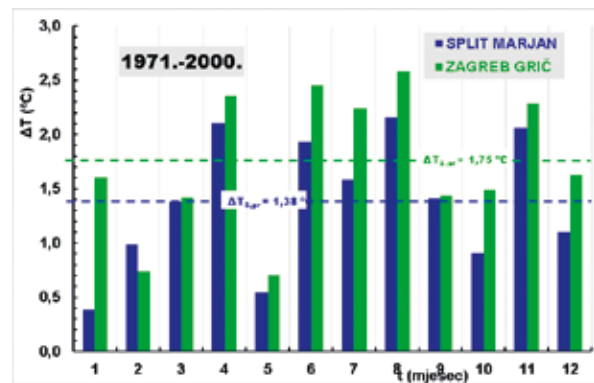
Slika 7: Histogrami mjesečnih razlika, \Delta T = T - T_{pr} , Split Marjana (modra boja) i Zagreb Griča (zeleno) u posljednjih deset godina (2011. - 2020.) u odnosu na drugo 30-godišnje razdoblje (1971. - 2000.)
