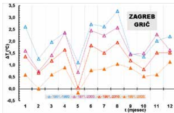
Slika 5: Grafički prikazi niza srednjih mjesečnih razlika, \Delta T = T - T_{pr} , za postaju Zagreb Grič u četiri 30-godišnja razdoblja
