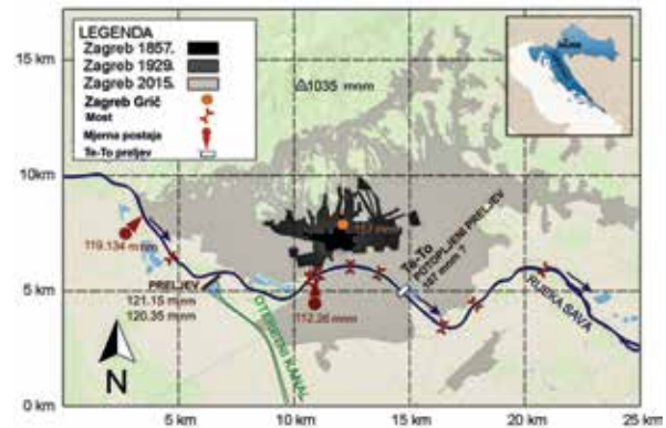
Slika 2: Karta s ucrtanim vodomjernim postajama Podused i Zagreb, preljevom Jankomir i oteretnim kanalom te položajem Te-To potopljenog preljeva (praga) i mostova na rijeci Savi u širem području Zagreba
